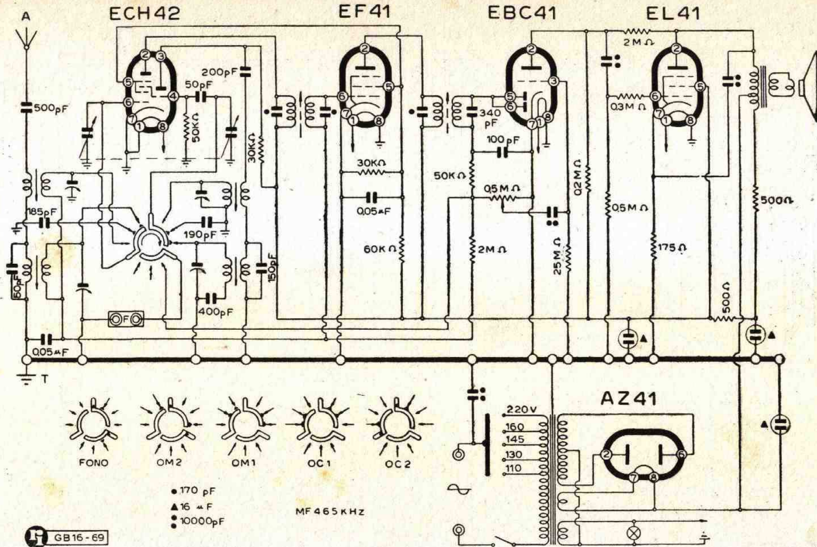
Lo schema elettrico del Mod. 510. La Voce del Padrone
